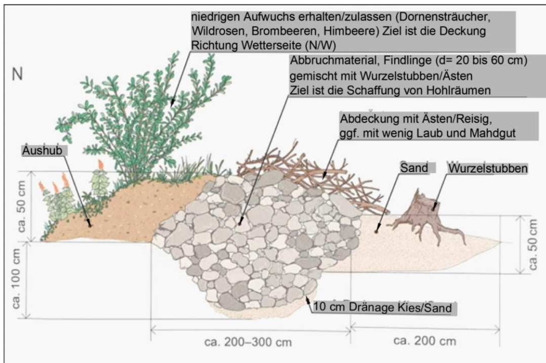
Abb. 17: Zauneidechsen - Winterquartier
