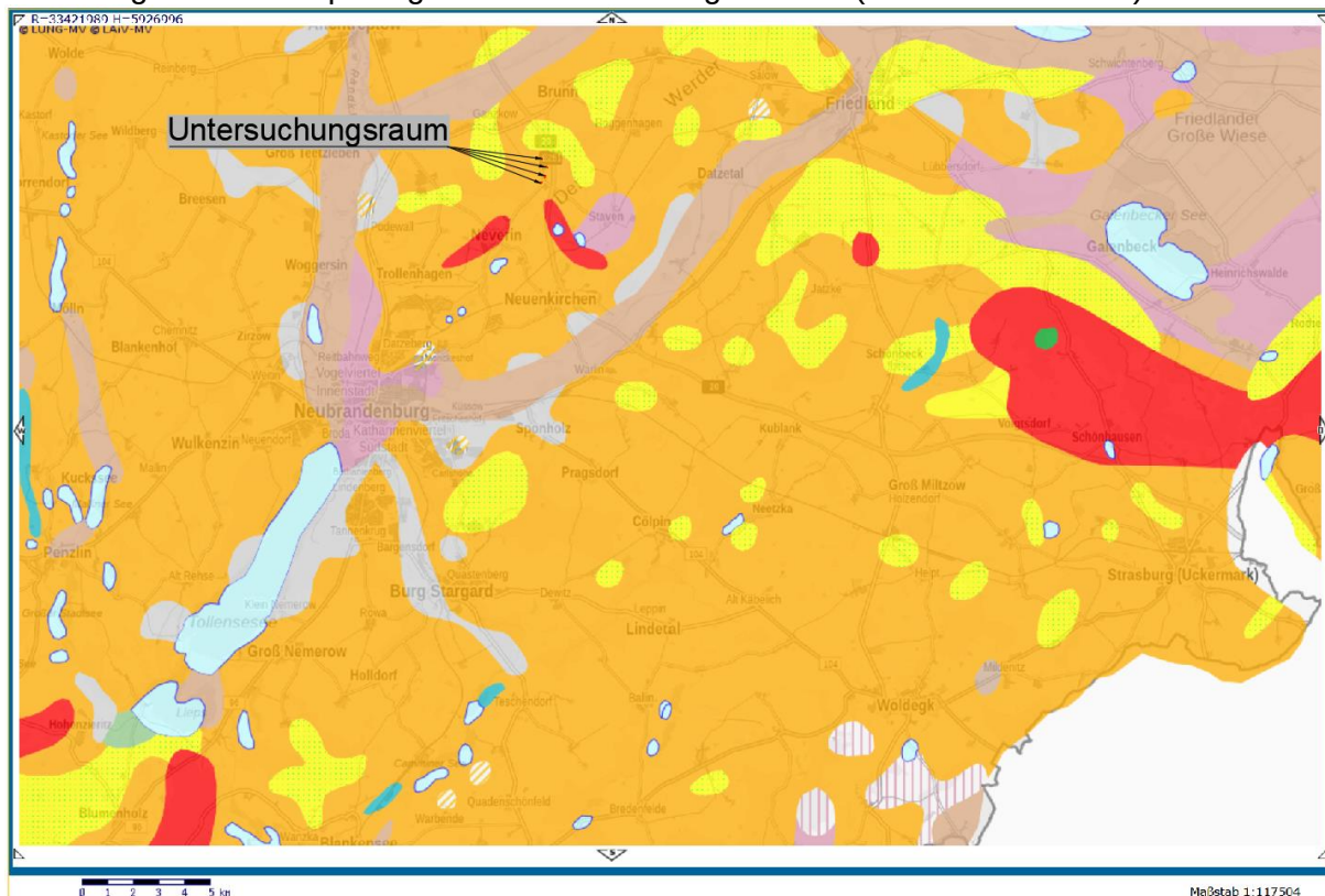
Abbildung 17: Geomorphologie des Untersuchungsraumes (© LAIV – MV 2022)
